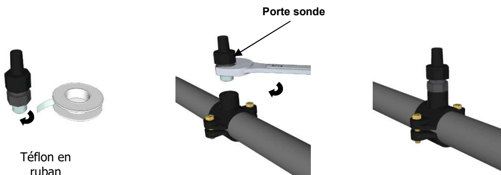
Porte sonde
